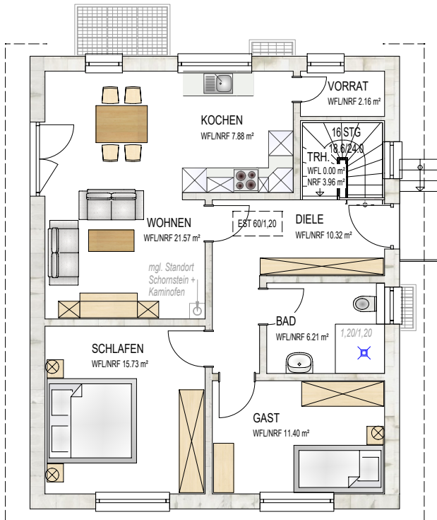
ERDGESCHOSS
